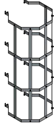
FRAMESET Güvenlik Kafesi H185 FRAMESET Safety Cage H185
